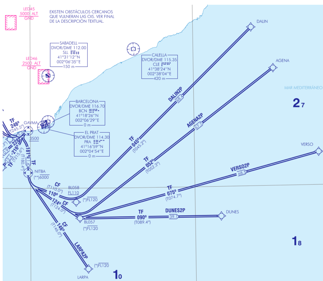
Figura 3.20: Extracto de SID P-RNAV de la RWY 25R de LEBL [Fig25].
