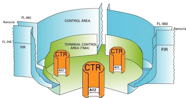
Figura 3.13: Sectorización de las zonas de control ATC [Fig16].
