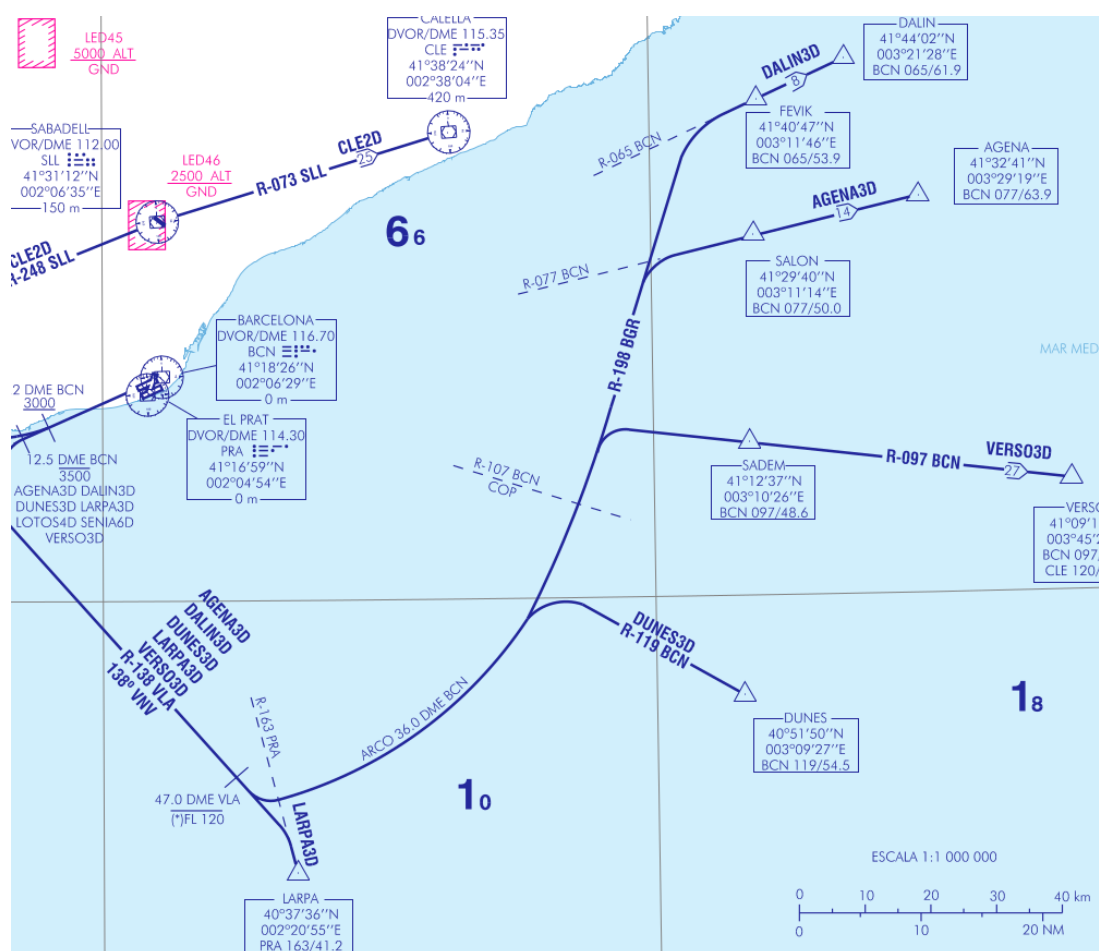
Figura 3.19: Extracto de SID convencional de la RWY 25R de LEBL [Fig25].
